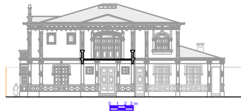
Elevation 02
